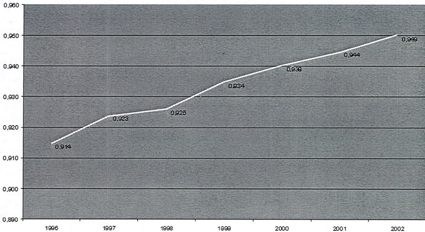
Gjennomsnitt HQ diagnose for hunder registrert 1996 - 2002
